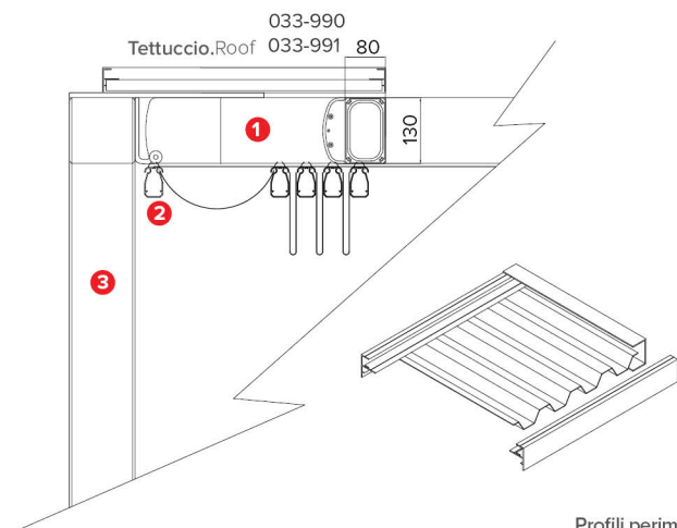
Dettaglio tettuccio . Roof detail
